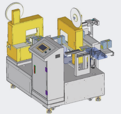
가로·세로 자동결속용 자동화라인 설계 예
